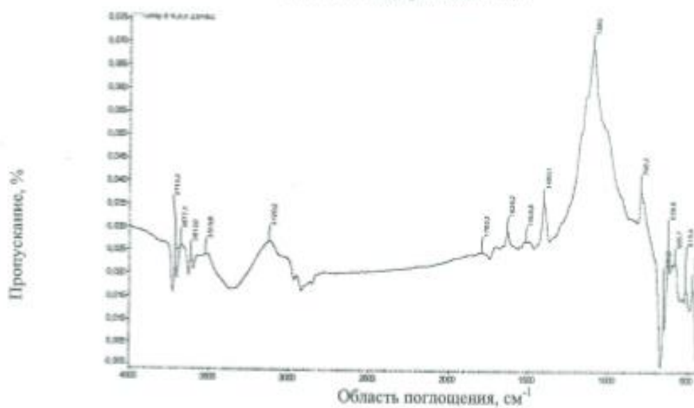
Рис. 4. ИК-спектр пирита FeS 2
