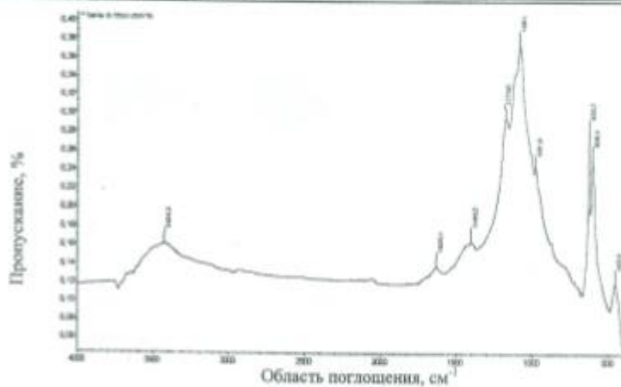
Рис. 3. ИК-спектр галенита PbS
